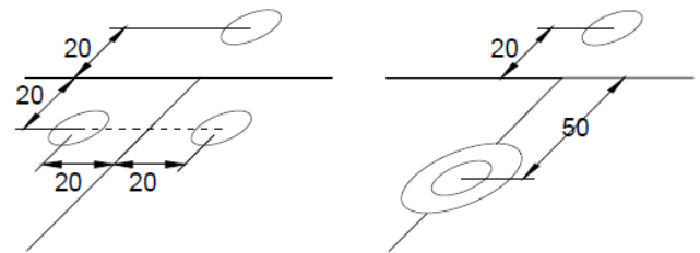
Distancias (en cm) a borde de panel de los tornillos con arandela 4,8 mm de diámetro y arandela de 40 mm de diámetro
