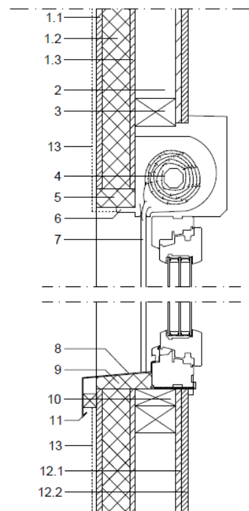
Figura 5.4: Encuentro tipo de fachada formada con paneles SATE y revestimiento interior COAT con carpintería y caja de persiana. Sección transversal vertical.
