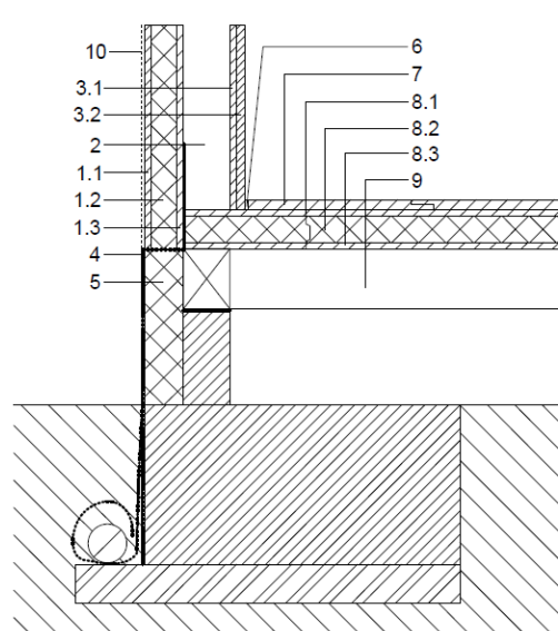
Figura 5.10: Encuentro tipo de fachada con paneles SATE y revestimiento interior COAT con forjado de sanitario. Sección transversal vertical.
