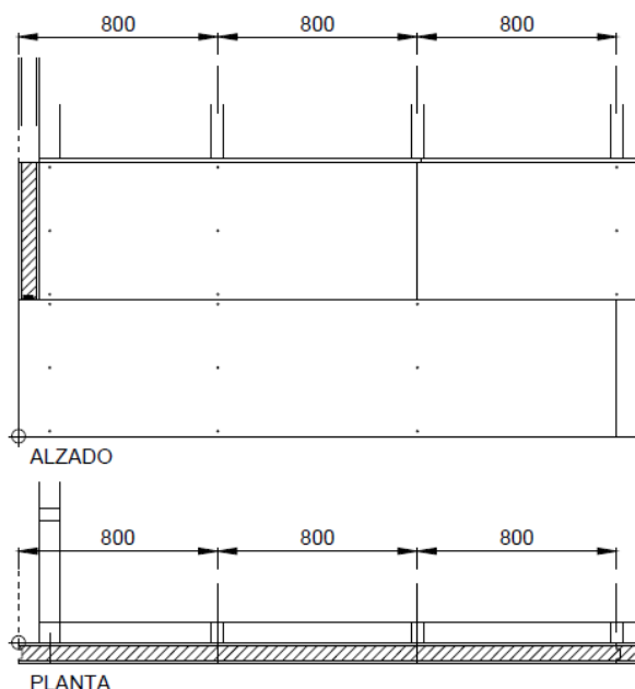
Figura 6.5: Colocación de la segunda hilada de paneles.
