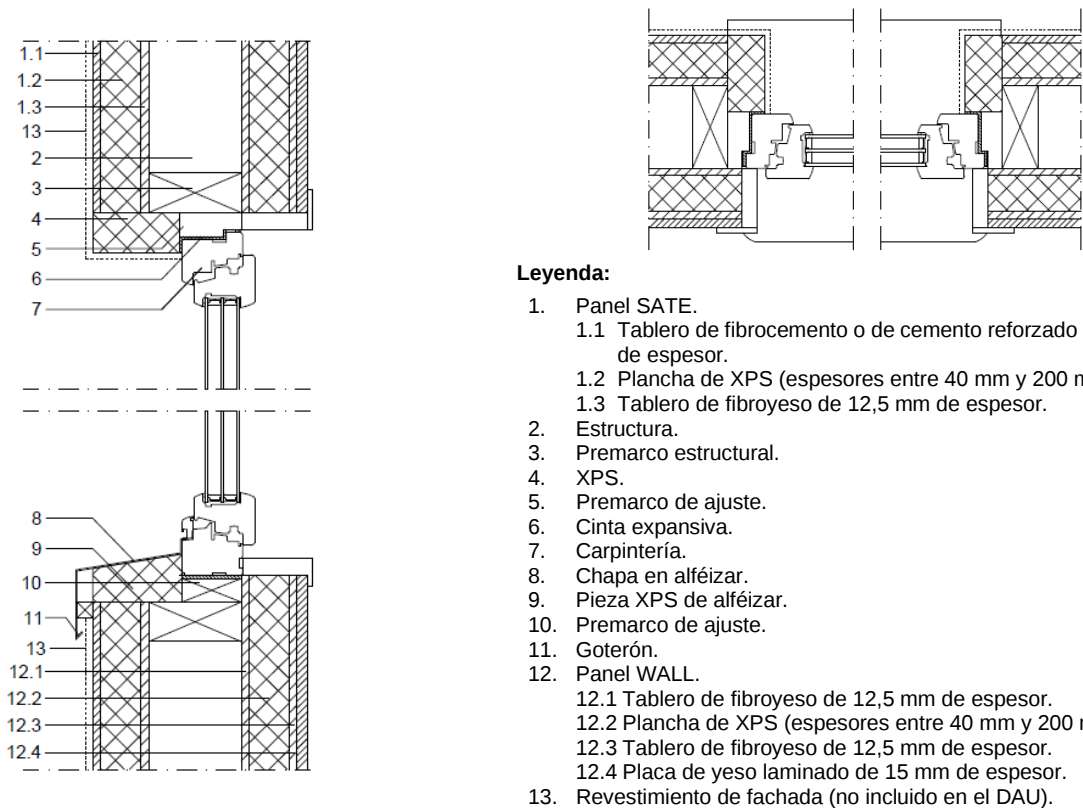
Figura 5.1: Encuentro tipo de fachada formada con paneles SATE y WALL con carpintería. Sección transversal horizontal y vertical.
