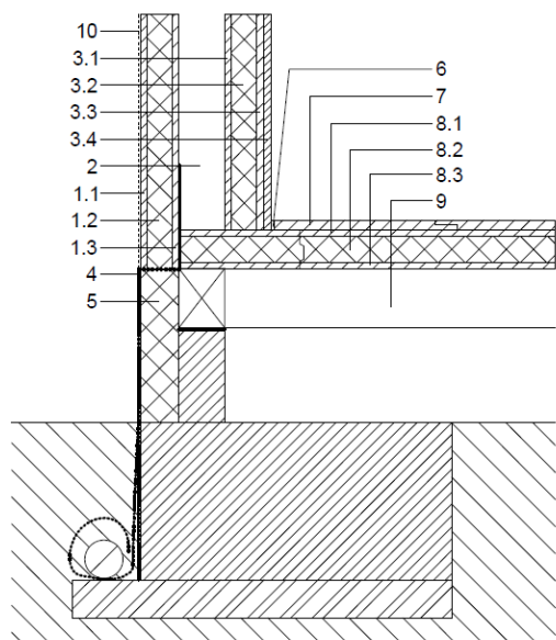
Figura 5.10: Encuentro tipo de fachada con paneles SATE y revestimiento interior COAT con forjado de sanitario. Sección transversal vertical.
