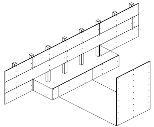
Figura 1.6: Montaje de Sistema Thermochip con revestimiento interior COAT.
