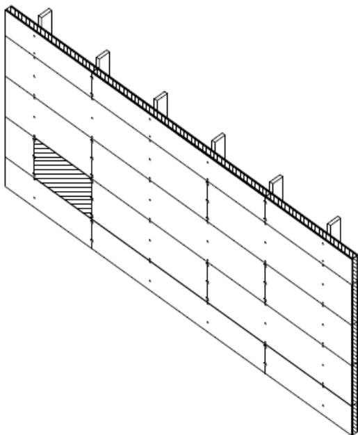
Figura 6.16 Reparación de daños severos en la cara del panel SATE.
