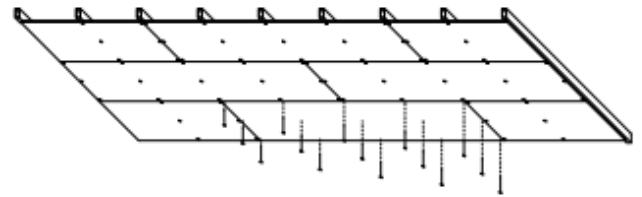
Figura 6.6: Disposición de tableros de fibroyeso sobre la estructura.
