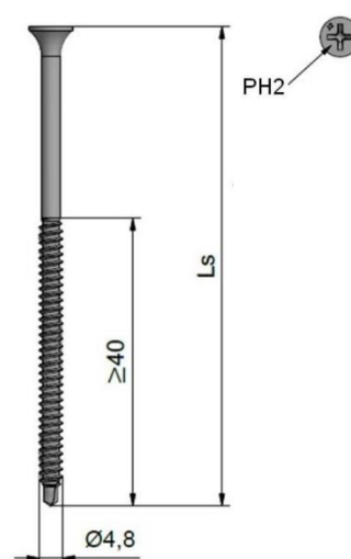
Figura 2.5: Tornillo sin arandela de 4,8 mm de diámetro.
